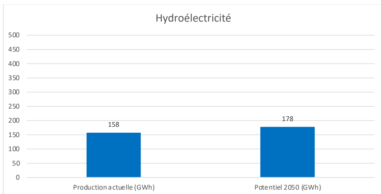
Figure 55 : Production hydroélectrique actuelle et potentielle
