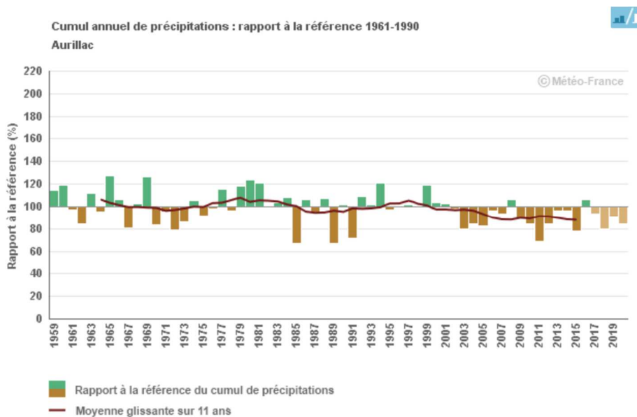
Figure 100 : Cumul annuel de précipitations par rapport à la référence 1961 - 1990 à Aurillac ; Source : Météo France / Climat HD
