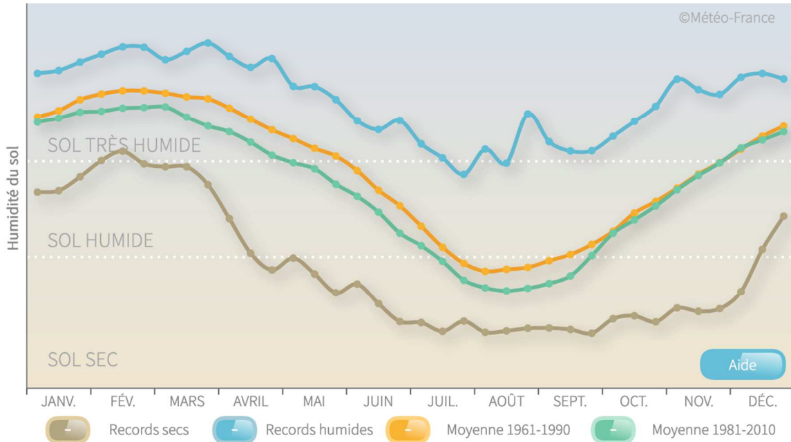
Figure 101 : Cycle annuel d'humidité des sols : moyenne et records ; Source : Météo France / Climat HD
