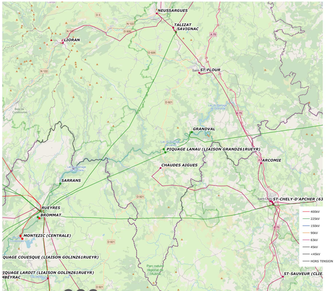
Figure 71 : Carte du réseau de transport sur le territoire de Saint-Flour Communauté. Source : rte-France.com
