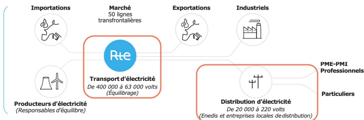
Figure 70 : Architecture du réseau électrique français, du plus haut niveau de tension (HTB3, 400 kV, au plus faible (BT, 400 V). Source : RTE.
