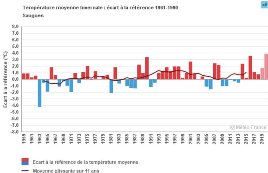
Figure 99 : Température moyenne annuelle (écart et référence 1961 - 1990) à Saugues ; Source : Météo France / Climat HD
