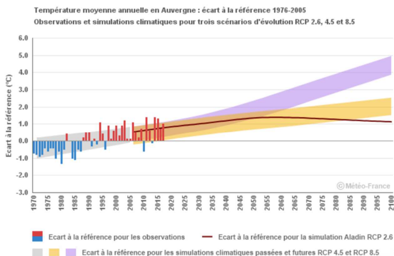
Figure 105 : Température annuelle en Auvergne : écart à la référence 1976 - 2005 pour 3 scénarii d'évolution RCP2.6, 4.5 et 8.5 ; Source : Météo France / Climat HD
